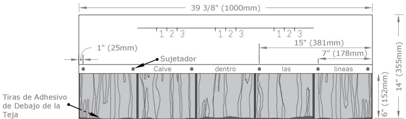
FIGURA 4 - Ubicación de Sujetador
